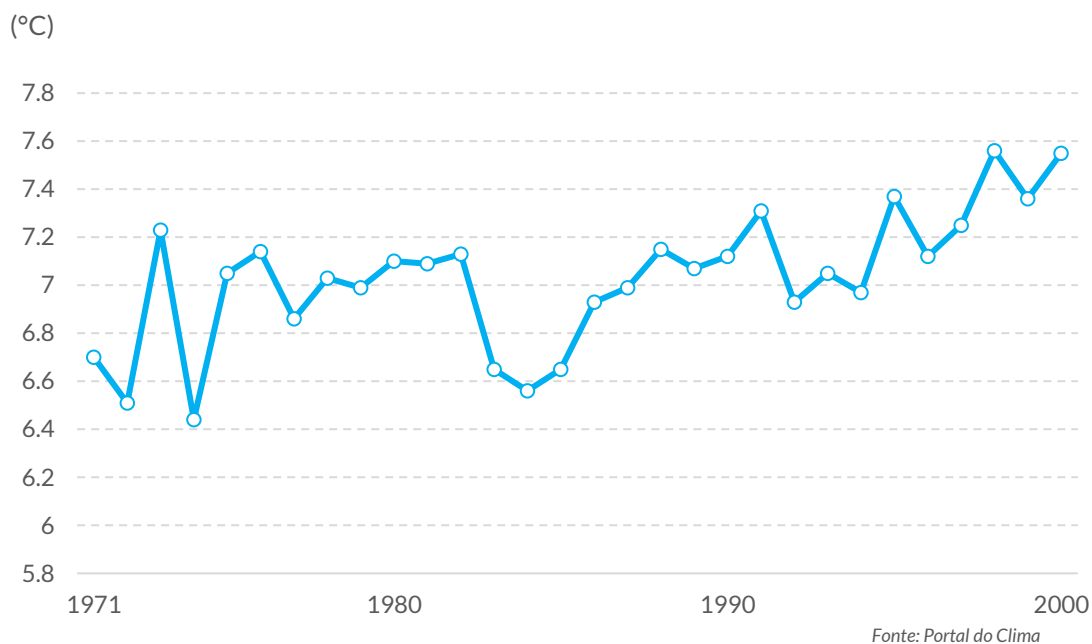
Gráfico 11. Histórico simulado da temperatura média mínima (°C) na região de Viseu Dão Lafões
