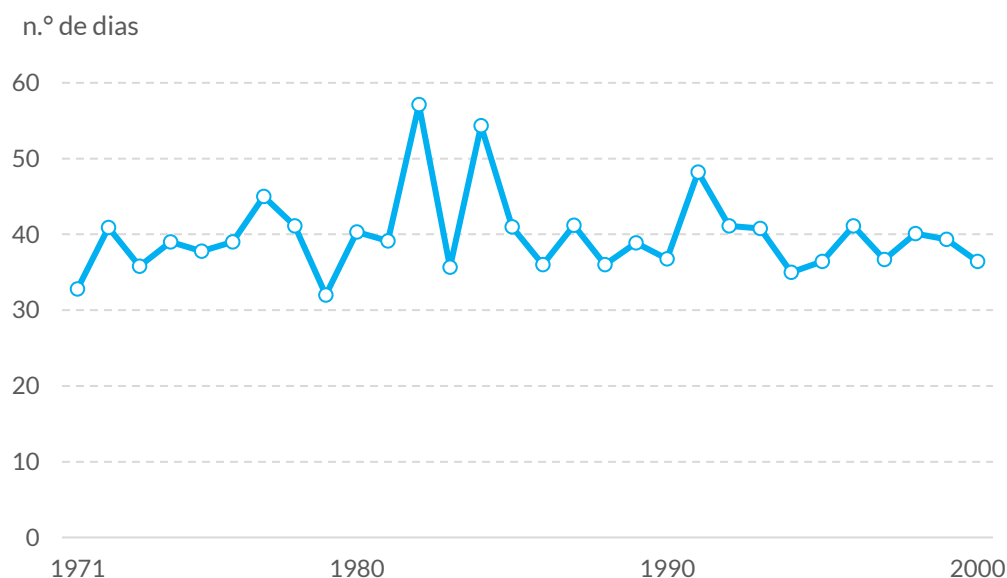
Gráfico 31. Histórico simulado de dias consecutivos sem chuva (n.º) na região de Viseu Dão Lafões
