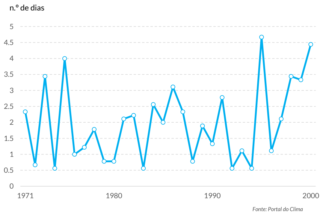
Gráfico 19. Histórico simulado de dias muito quentes (n.º) na região de Viseu Dão Lafões
