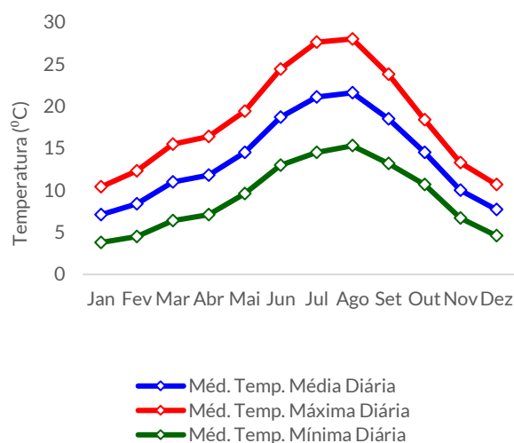
Gráfico 8. Valores de temperatura, 1981-2010, em Viseu
