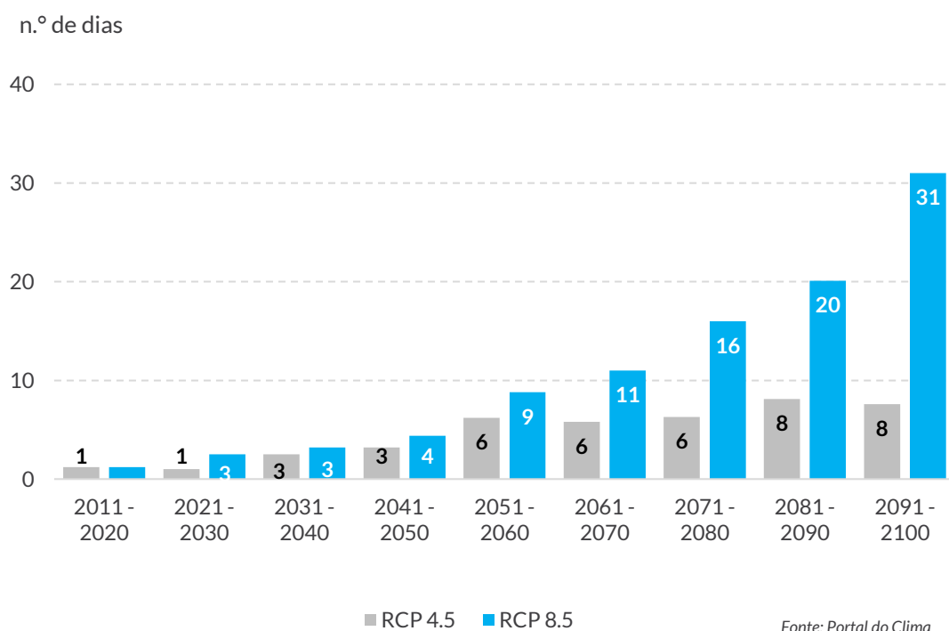
Gráfico 20. Anomalias de dias muito quentes (n.º) na região de Viseu Dão Lafões
