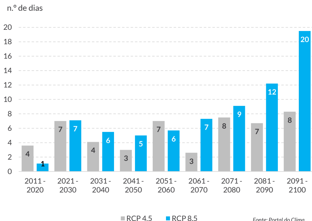
Gráfico 32. Anomalias de dias consecutivos sem chuva (n.º) na região de Viseu Dão Lafões
