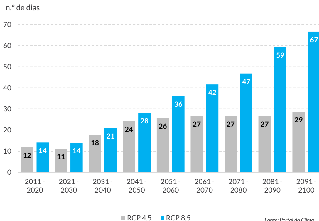
Gráfico 18. Anomalias de dias de verão (n.º) na região de Viseu Dão Lafões
