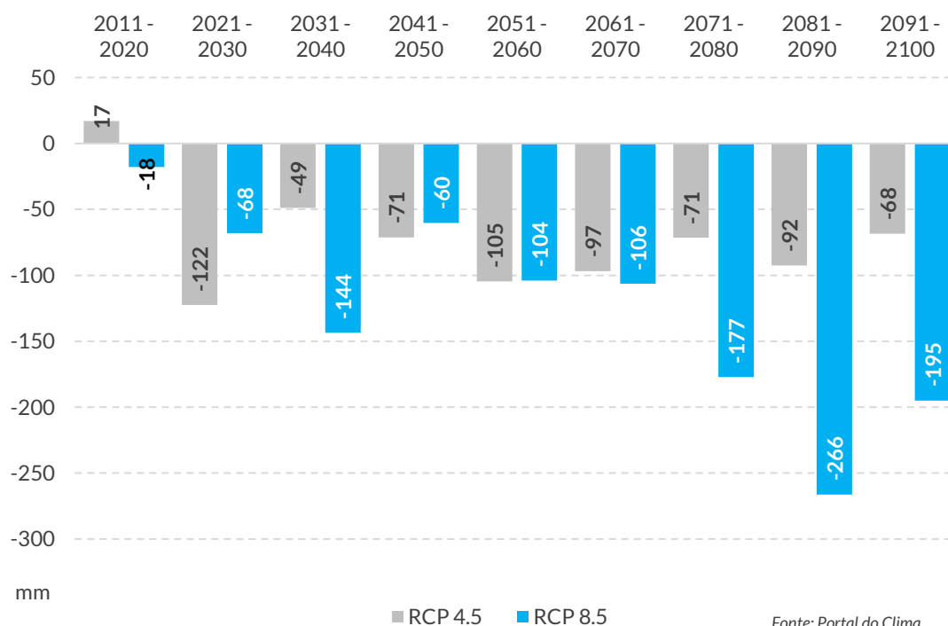
Gráfico 24. Anomalias de precipitação média acumulada (mm) na região de Viseu Dão Lafões
