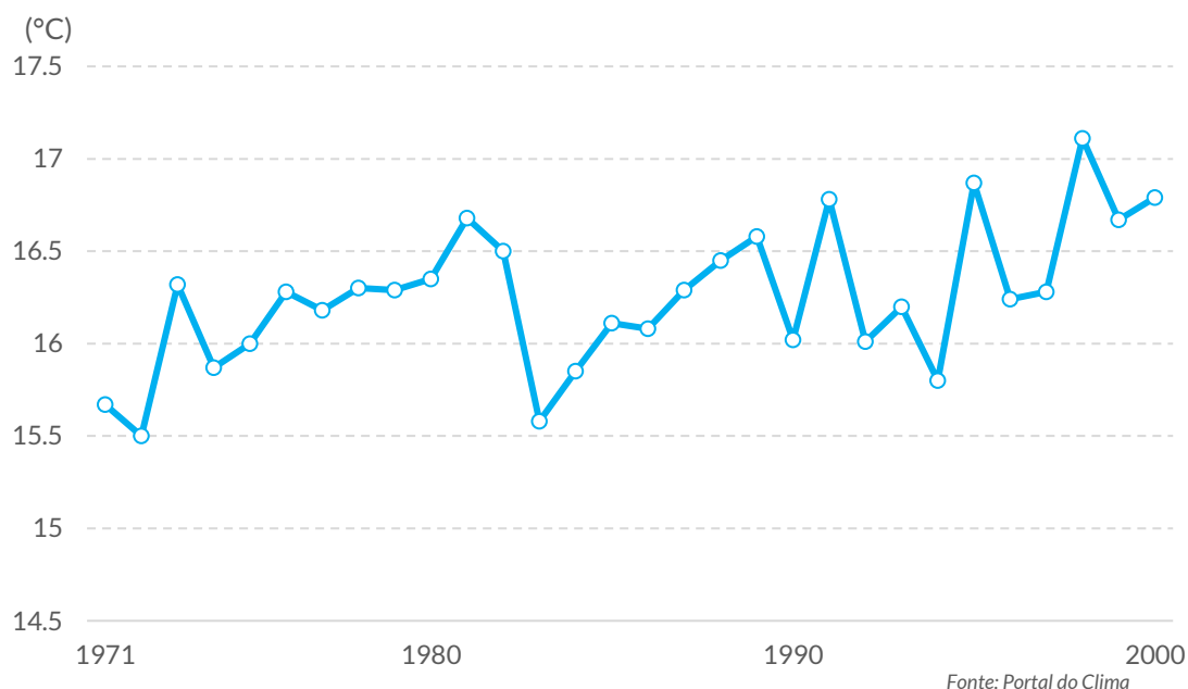
Gráfico 15. Histórico simulado da temperatura média máxima (°C) na região de Viseu Dão Lafões
