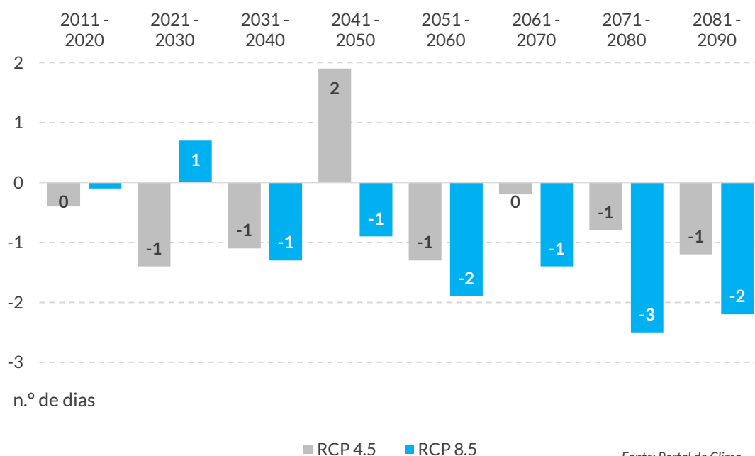
Gráfico 34. Anomalias de dias consecutivos com chuva (n.º) na região de Viseu Dão Lafões
