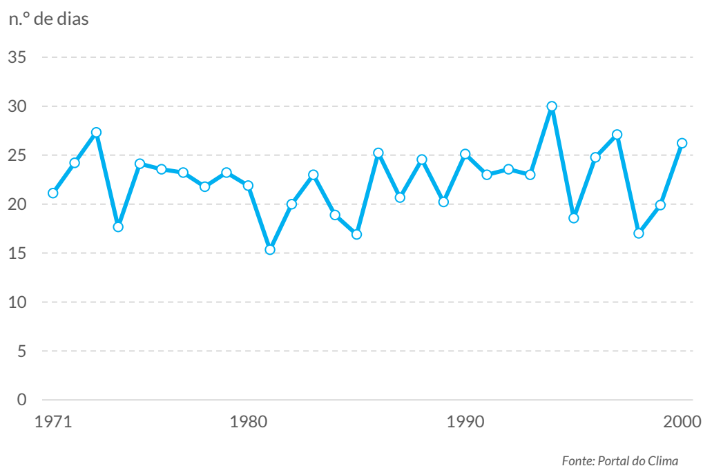
Gráfico 29. Histórico simulado de dias com precipitação superior a 20mm (n.º) na região de Viseu Dão Lafões
