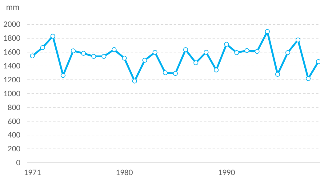
Gráfico 23. Histórico simulado de precipitação média acumulada (mm) na região de Viseu Dão Lafões
