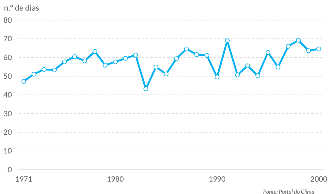
Gráfico 17. Histórico simulado de dias de verão (n.º) na região de Viseu Dão Lafões
